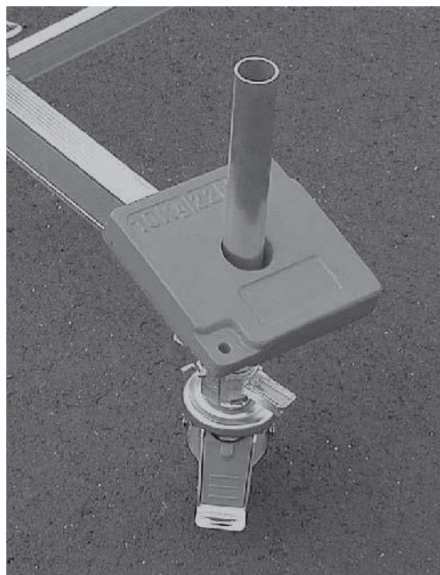
Balastowanie stabilizatora
